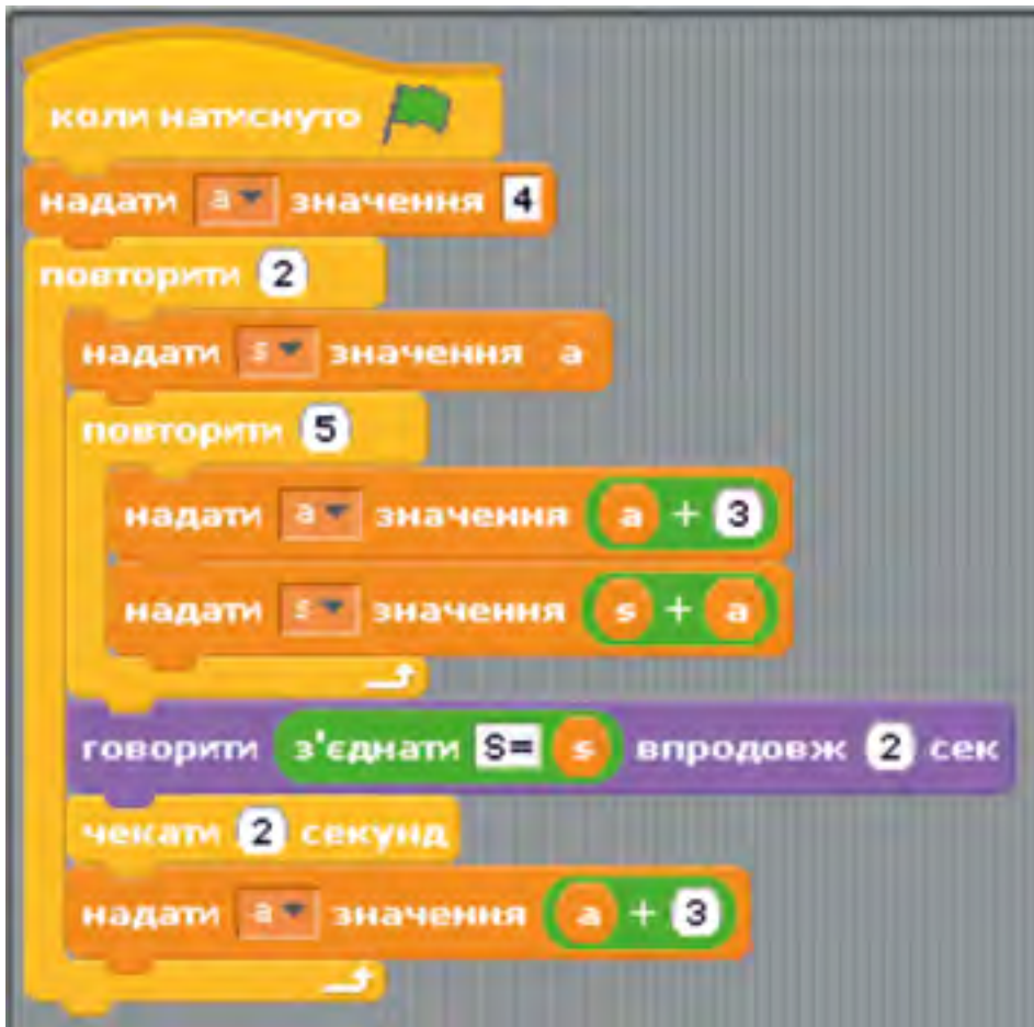
Рис. 5.3. Програма обчислення суми послідовності чисел
