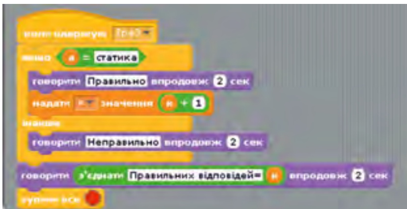
Рис. 5.8. Програма 2 для об'єкта з іменем Гра
