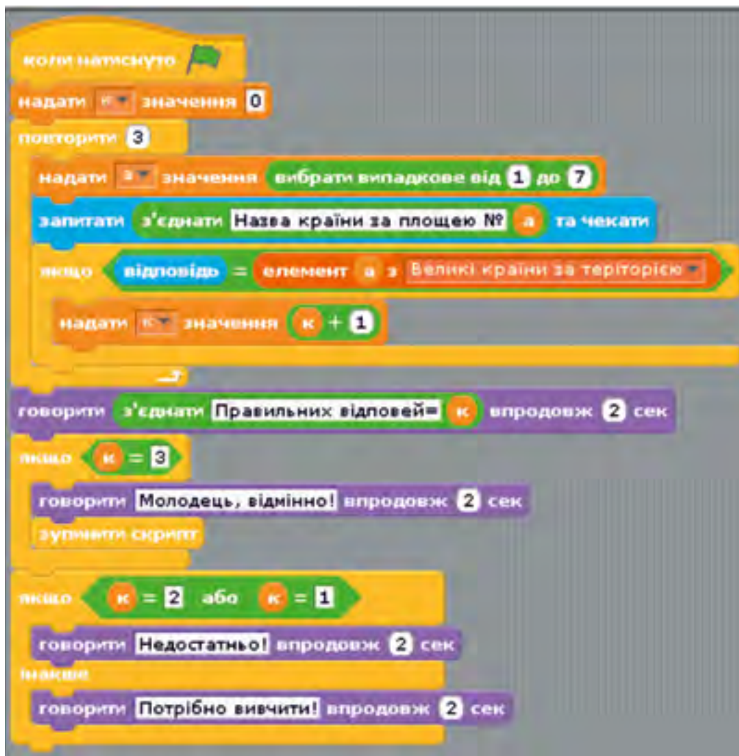
Рис. 6.2. Програма перевірки знань учнів із географії
