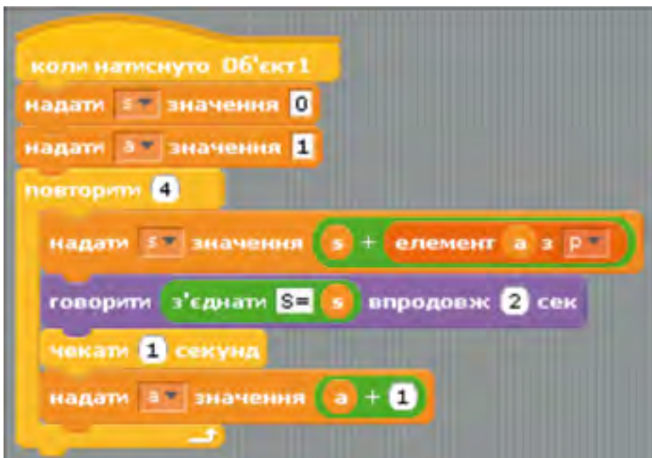
Рис. 3.63. Програма для самостійного аналізу
