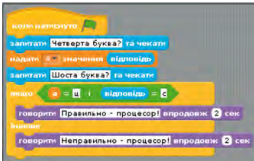
Рис. 3.75. Програма відгадування слова
