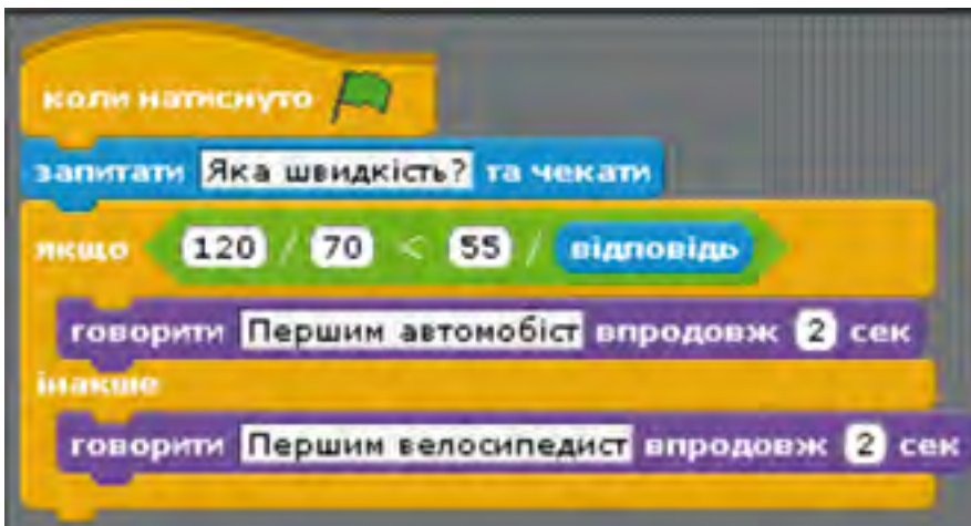
Рис. 3.74. Програма для формулювання умови задачі
