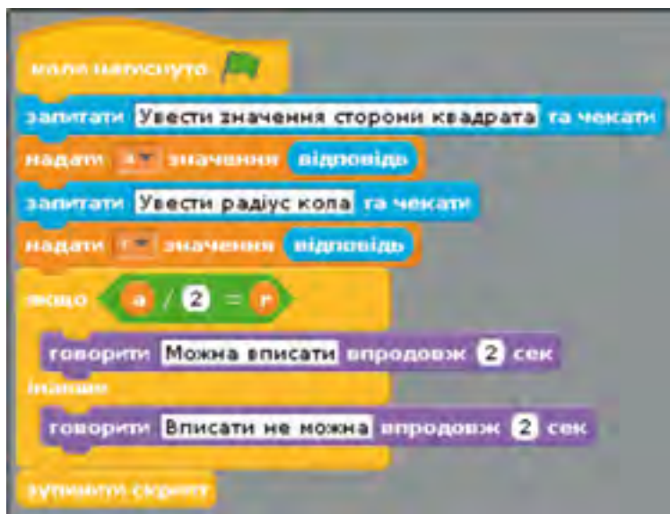
Рис. 3.66. Програма аналізу можливості вписати коло у квадрат
