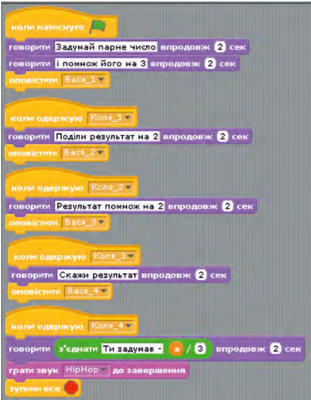
Рис. 5.4. Програми для об'єкта з іменем Коля
