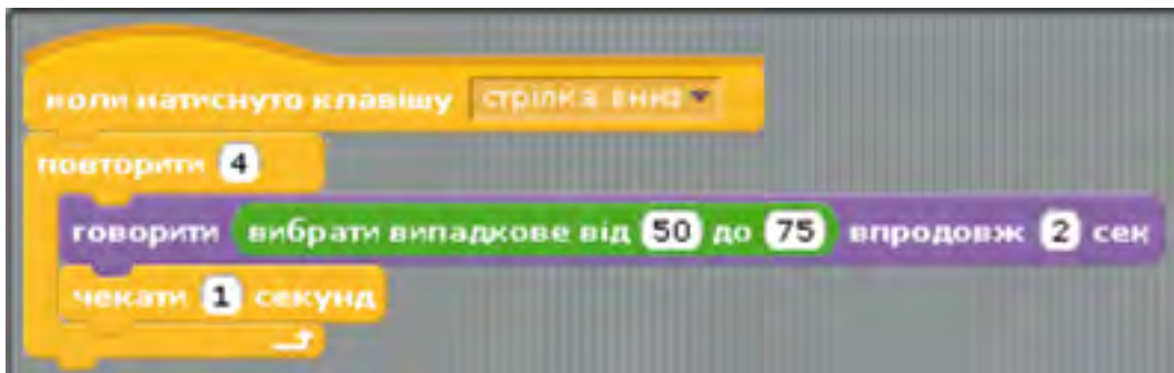
Рис. 3.44. Програма генерування випадкових чисел
