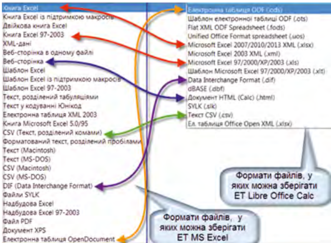
Рис. 4.6. Формати, в яких можуть бути збережені документи, що містять електронні таблиці (ліворуч – MS Excel, праворуч – Libre Office Calc)
