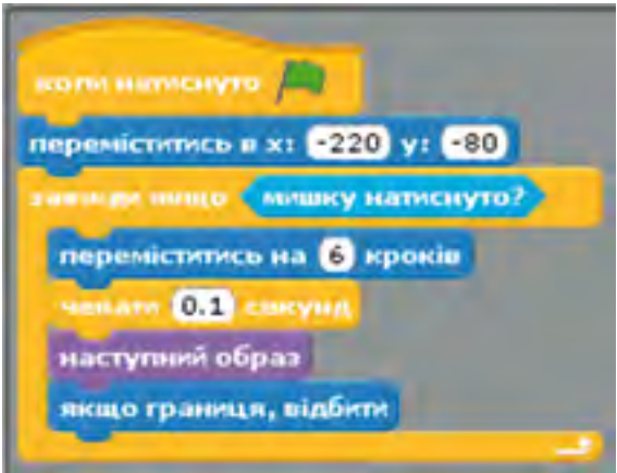
Рис. 3.78. Програма моделювання руху об'єкта boy4-walking
