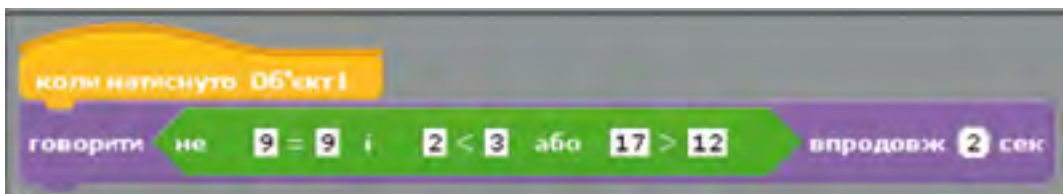
Рис. 3.39. Програма з логічним виразом
