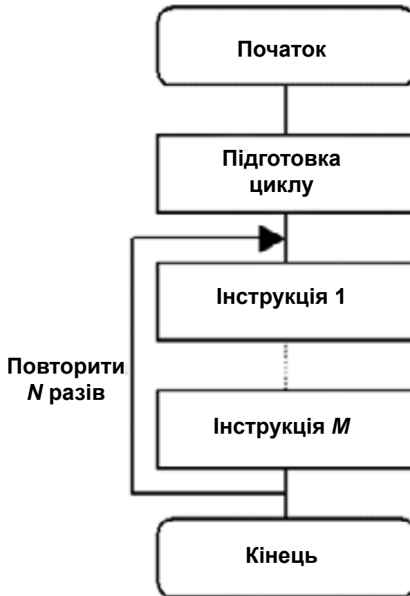
Рис. 3.17. Загальна структура алгоритму з повторенням
