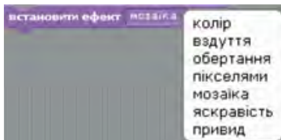
Рис. 3.46. Зарезервовані рядкові константи команди встановити ефект
