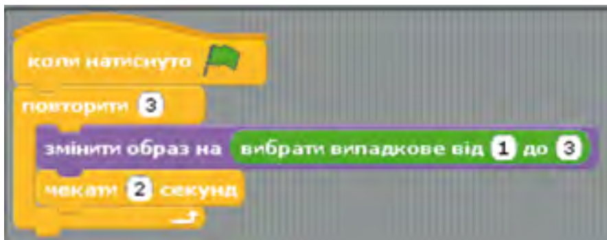
Рис. 3.45. Програма вибору випадкового образу
