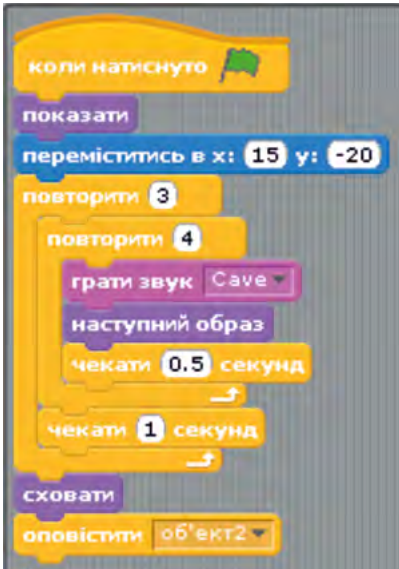
Рис. 6.3. Програма для об'єкта ballerina
