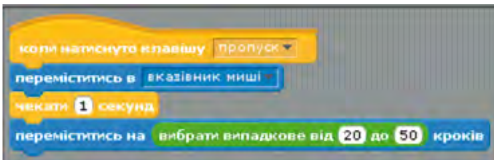
Рис. 3.33. Програма переміщення об'єкта на випадкову відстань
