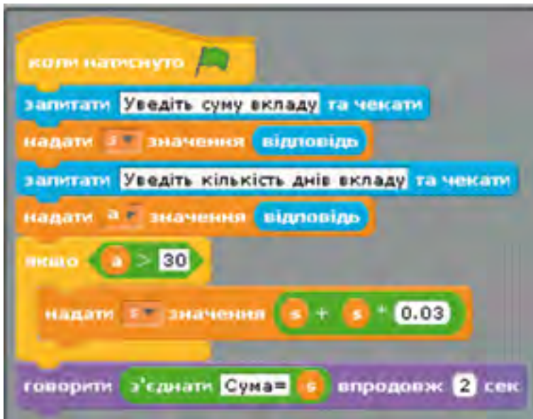
Рис. 3.69. Програма визначення суми внеску
