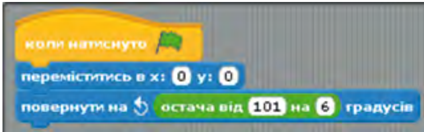
Рис. 3.32. Програма зміни напрямку руху об'єкта
