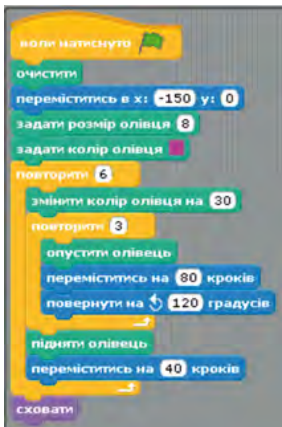
Рис. 3.84. Програма моделювання орнаменту
