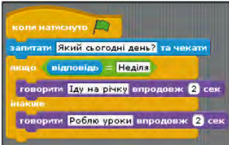
Рис. 3.73. Програма моделювання розмови Сашка і Каті
