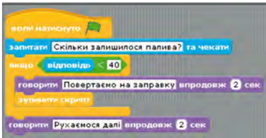
Рис. 3.70. Програма моделювання дій водія автомобіля
