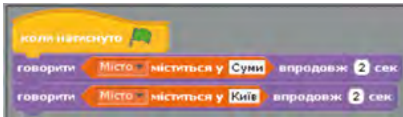
Рис. 3.59. Програма аналізу змісту списку
