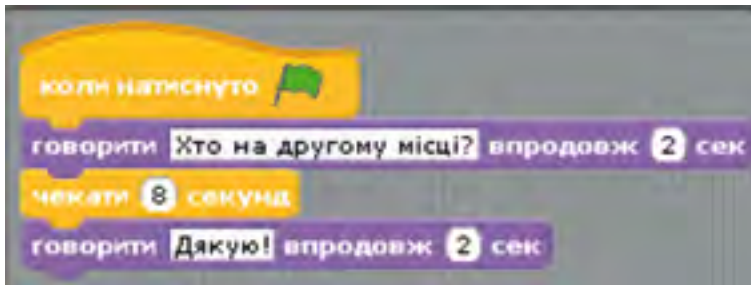
Рис. 3.56. Програма, що реалізує розмову Сергія
