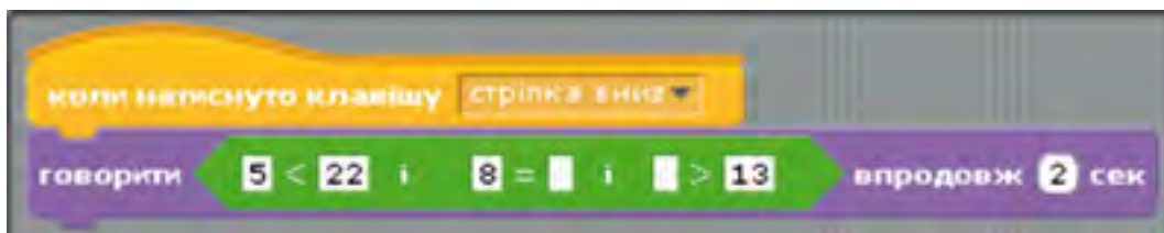
Рис. 3.40. Незавершена програма з логічним виразом
