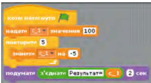
Рис. 3.58. Програма зміни значення змінної
