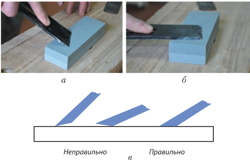
Рис. 55. Налагоджування ножа
