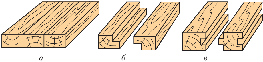
Рис. 61. Сп'ювання деталей: a – встик; б – в четверть; в – у шпунт і гребінь
