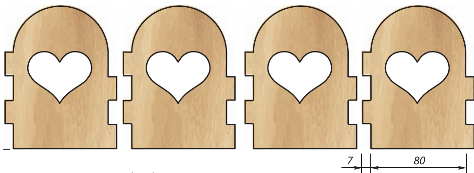
Бічні стінки виробу (фанера завтовшки 7 мм)
