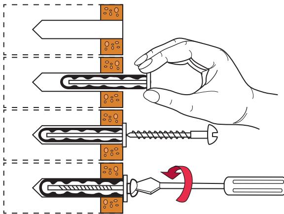
Рис. 114. Кріплення дюбеля
