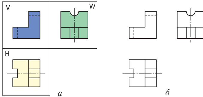
Рис. 34. Кресленник трьох проекцій: а – прямокутні проєкції предмета; б – кресленник
