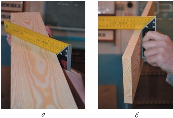
Рис. 60. Перевірка якості стругання: а – пласти; б – крайки (канта)
