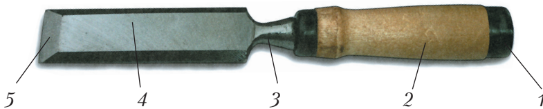
Рис. 68. Долото: 1 – кільце; 2 – ручка; 3 – шийка; 4 – різець; 5 – фаска
