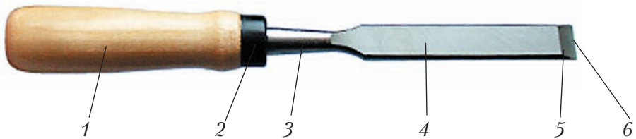
Рис. 69. Стамеска:
