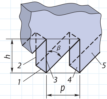
Рис. 46. Елементи зубців ножівки: 1 – передня різальна крайка; 2, 3 – бічні крайки; 4 – передня грань; 5 – задня грань
