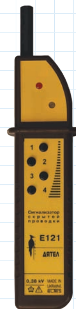
Рис. 112. Сигналізатор прихованої проводки E121 «Дятел». З його допомогою можна виявити електричні кабелі під штукатуркою завтовшки 5–7 см
