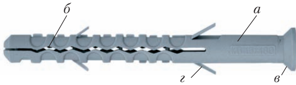
Рис. 105. Дюбель: а – нерозпірна частина, б – розпірна частина; в – манжета; г – вусяки
