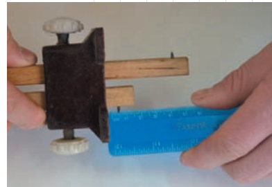
Рис. 42. Розмічання рейсмусом
