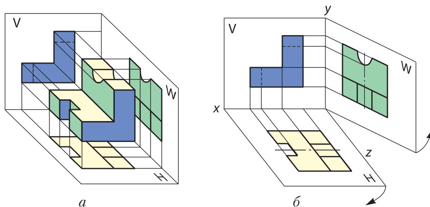
Рис. 33. Проєціювання на три площини проєкцій: a – проєкції предмета на площинах V , H і W ; б – побудова кресленика предмета
