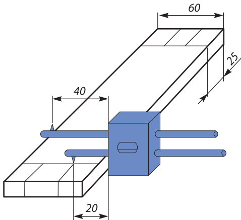
Рис. 65. Розмічання шипа
