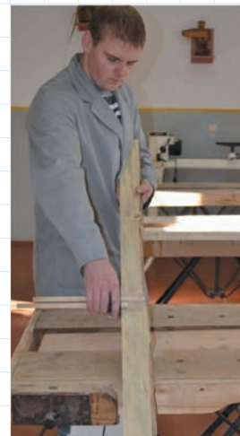
Рис. 44. Розмічання рейсмусом для стругання крайки
