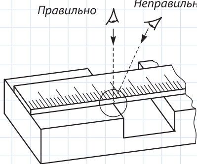
Рис. 39. Розмічання лінійкою
