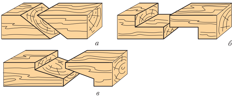
Рис. 62. З'єднання деталей зрощуванням: a – накладка; б – накладка впівдерева; в – накладка косим зрізом (коса фуга)
