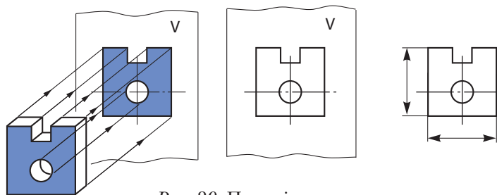
Рис. 29. Проєціювання на одну площину проєкцій
