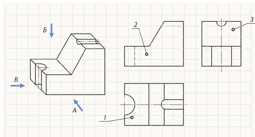
Рис. 35. Кутник
