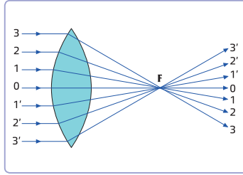
Мал. 56. Лінза лупи збирає паралельні промені в точці F — у фокусі
