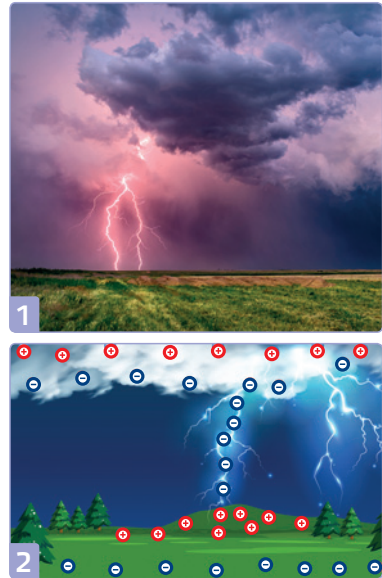
Мал. 29. Блискавки, що вдаряють у землю
