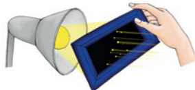
Модель сузір'я
