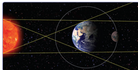
Мал. 95. Схема місячного затемнення
