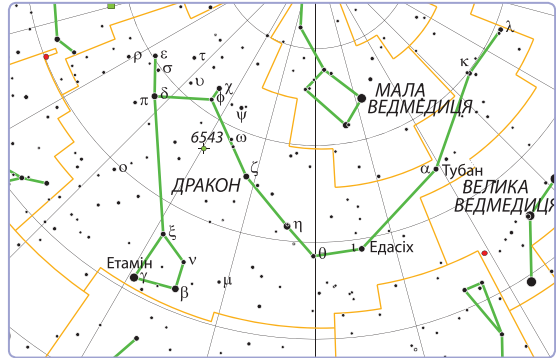
Мал. 145. Сузір'я зоряного неба
