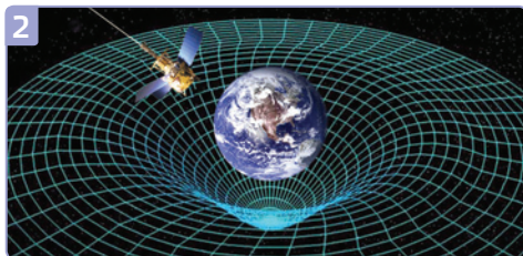
Мал. 84. Викривлення простору: 1 — Сонце, Земля і Місяць; 2 — Земля і супутник
