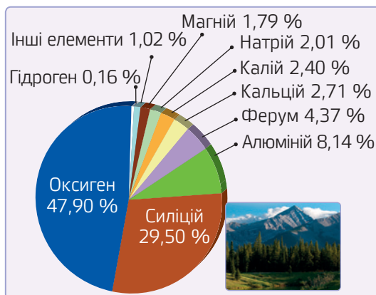
Мал. 68. Хімічний склад земної кори
