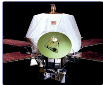
Мал. 157. Космічний апарат «Марінер-9»
