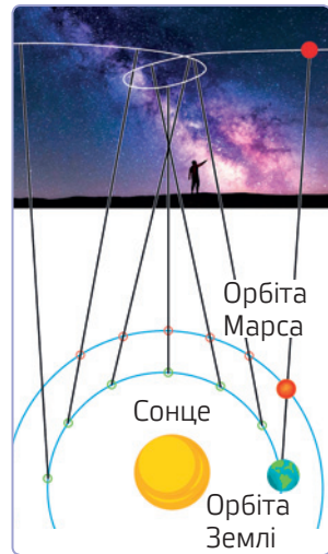
Мал. 181. Чому планети «петляють» на небі
