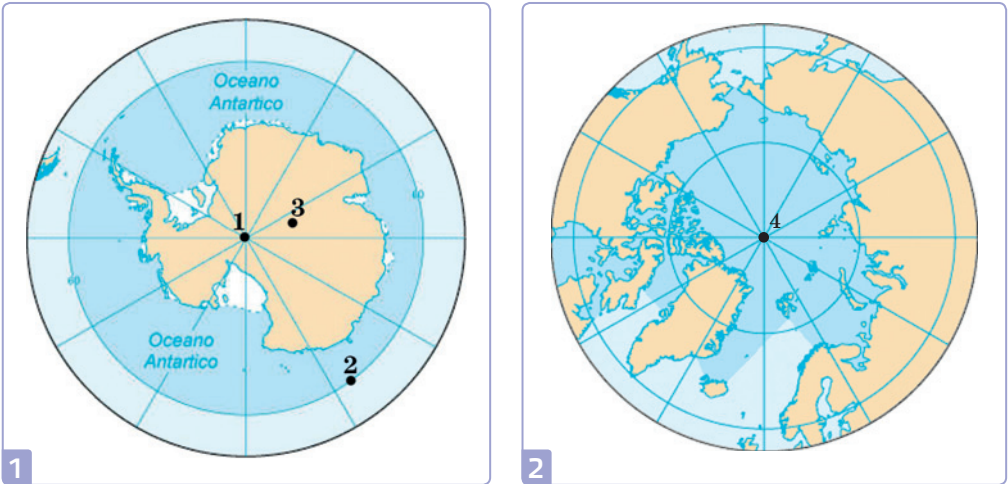
Мал. 241. Приполярні зони: 1 — Південний полюс, 2 — південний магнітний полюс, 3 — південний полюс недосяжності, 4 — Північний полюс
