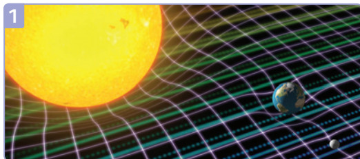
Мал. 84. Викривлення простору: 1 — Сонце, Земля і Місяць; 2 — Земля і супутник
