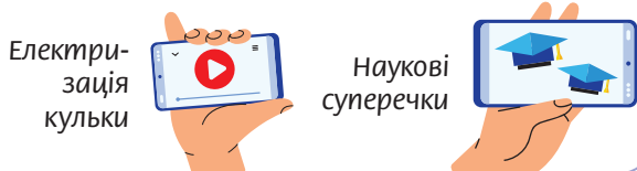
Мал. 25. Взаємодія однойменних та різнойменних зарядів
