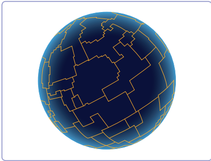
Мал. 144. Небесну сферу поділено на 88 ділянок
