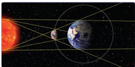
Мал. 93. Схема сонячного затемнення
