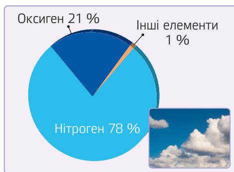
Мал. 70. Хімічний склад атмосфери
