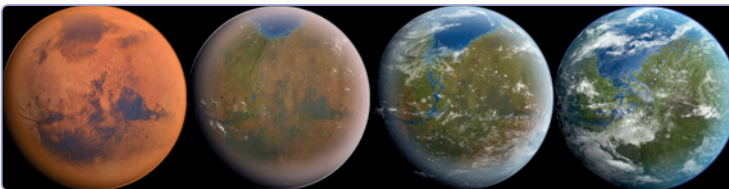
Мал. 179. Етапи тераформування Марса. Ілюстрація
