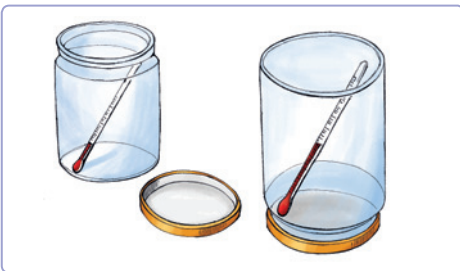
Мал. 153. Модель парникового ефекту
