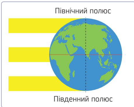
Мал. 89. Поблизу полюсів на Землю потрапляє менше сонячної енергії
