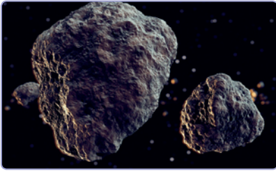
Мал. 166. Метеороїди
