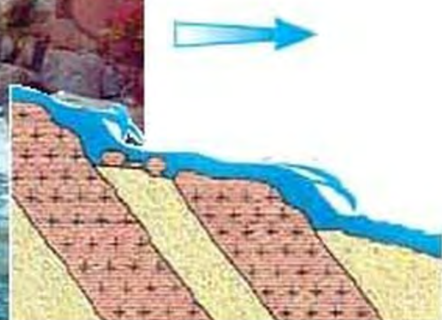
Схема утворення порогів
