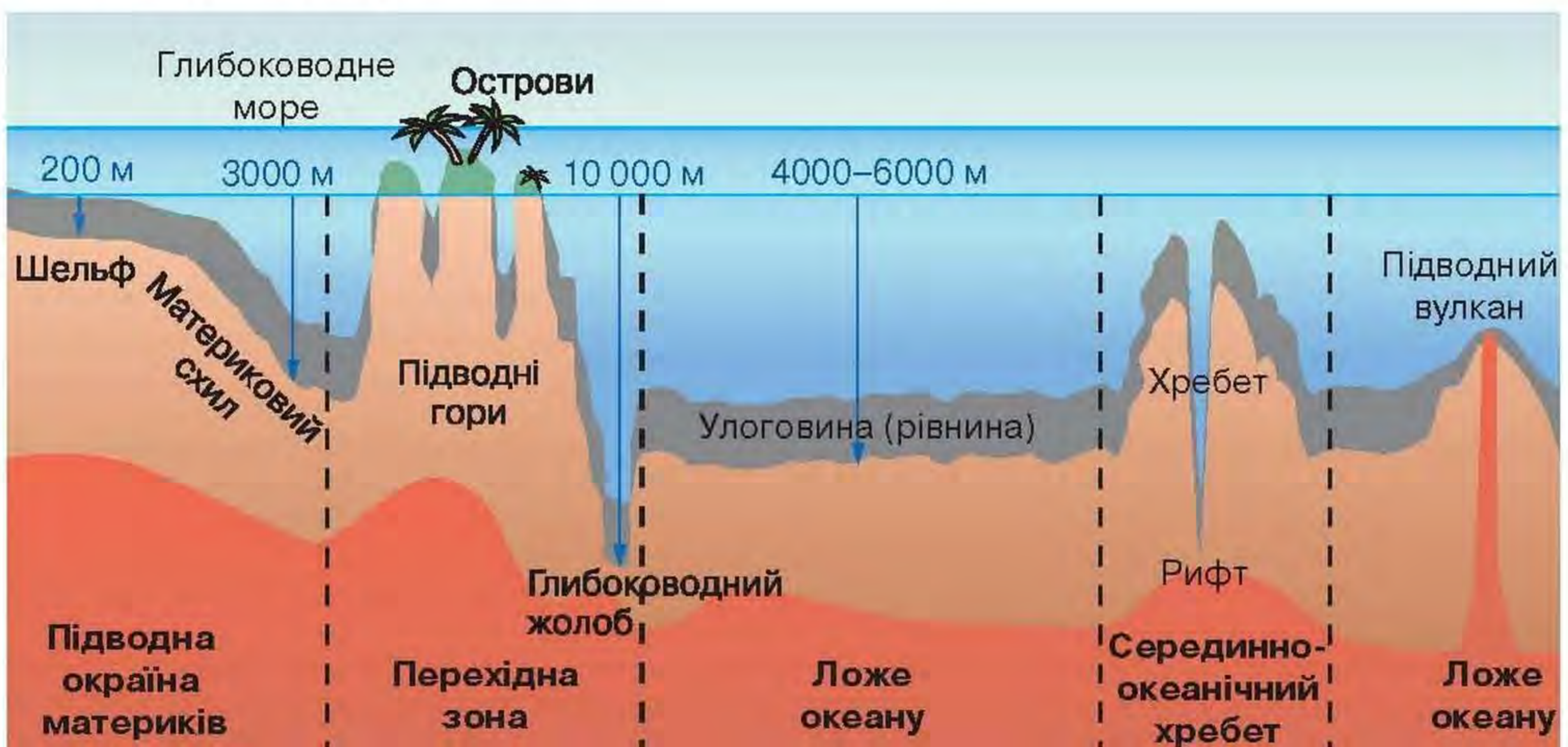
Мал. 113. Схема рельєфу дна океану
