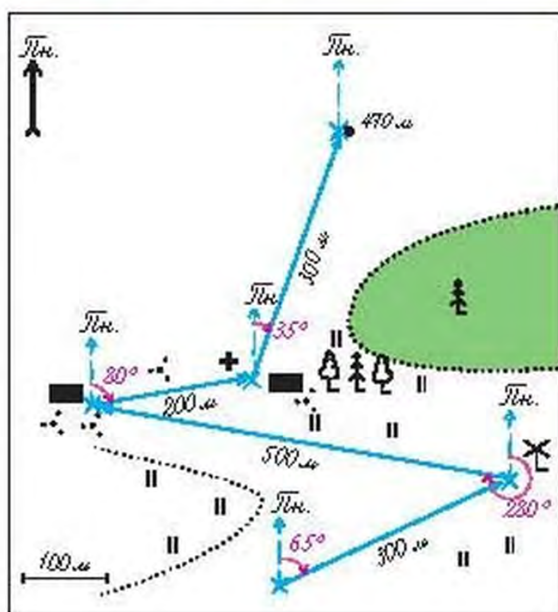
Мал. 46. Окомірне маршрутне знімання місцевості
