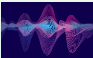
Зображення звукової хвилі
