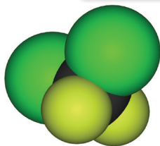
Рис. А. Молекула дифлуоро-дихлорометану (фреону R-12).
