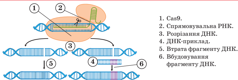
Рис. 43.4. Схема генної модифікації заснована на системі CRISPR/Cas9
