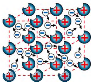
Рис. 42. Схема утворення металічного зв'язку
