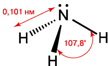
Рис. 14. Схема будови молекули амоніаку
