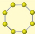
Ромбічна
