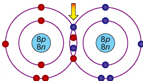
Рис. 12. Схема утворення двох спільних електронних пар у молекулі кисню
