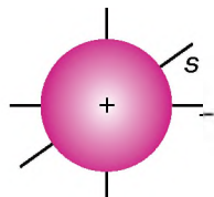
Рис. 2. Форма s -орбіталі та розміщення її в просторі
