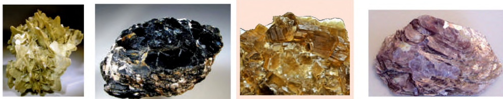
Рис. 57. Види слюди: а — мусковіт; б — біотит; в — флогопіт; г — лепідоліт
