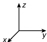
Рис. 1. Вісь координат
