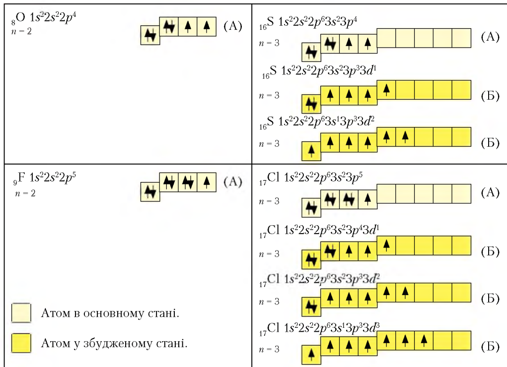
Рис. 9. Розміщення електронів по орбіталях в атомах неметалічних елементів 2 та 3 періодів в основному (А) та збудженому (Б) станах
