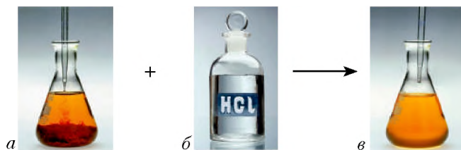
Рис. 39. Розчинення ферум(III) гідроксиду під час взаємодії з хлоридною кислотою: а – ферум(III) гідроксид; б – хлоридна кислота; в – прозорий розчин ферум(III) хлориду
