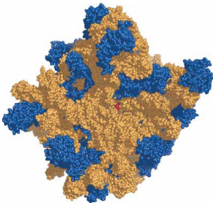
Мал. 18.7. Структура великої субдиниці рибосоми: жовтим кольором позначено рРНК, синім – білки, червоним – активний центр
