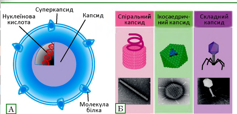
Рис. 12.1. Будова вірусів
