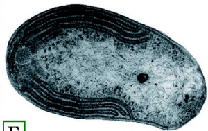
Рис. 6.4. Нітрифікатори ґрунту
