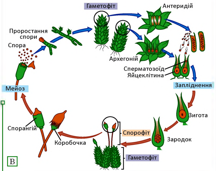
Рис. 8.3. Мохоподібні
