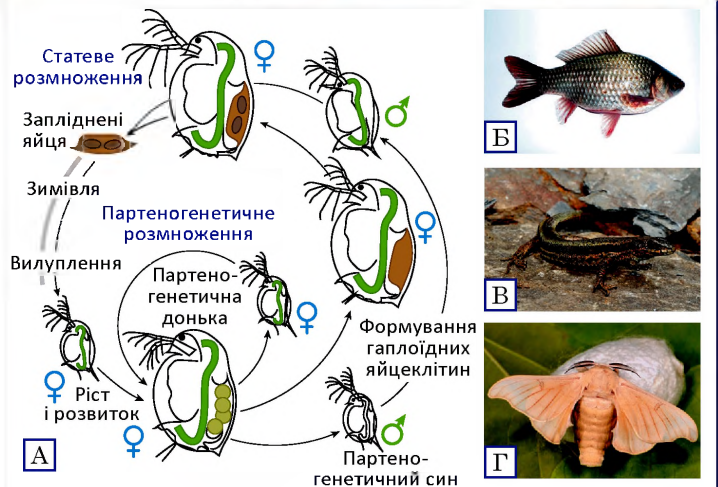
Рис. 39.4. Партеногенез
