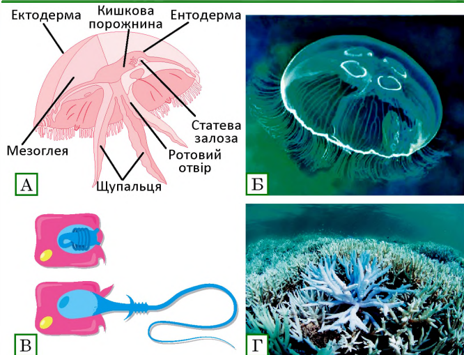
Рис. 10.2. Кишковопорожнинні
