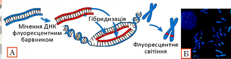
Рис. 37.5. Флуоресцентна гібридизація
