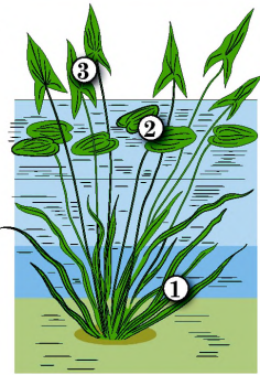
Рис. 34.3. Стрiлця
