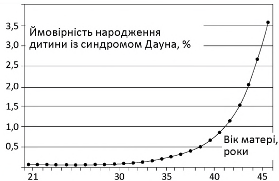
Рис. 36.3. Синдром Дауна
