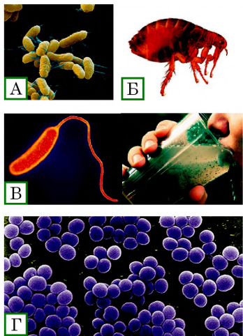
Рис. 6.8.
