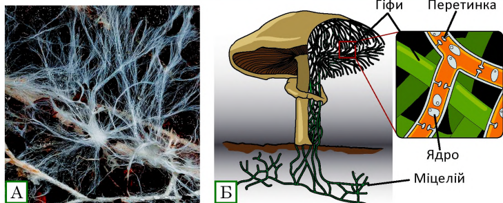
Рис. 9.1. Будова грибів
