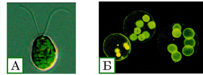
Рис. 7.8. Зелені водорості
