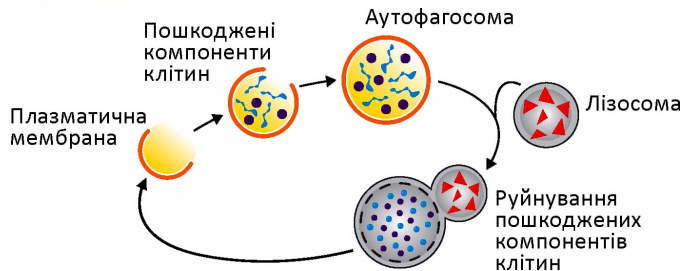
Рис. 43.5. Процес аутофагії
