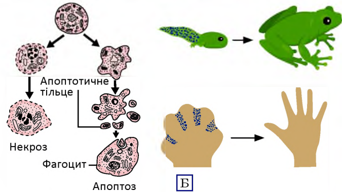
Рис. 45.2. Клітинна смерть
