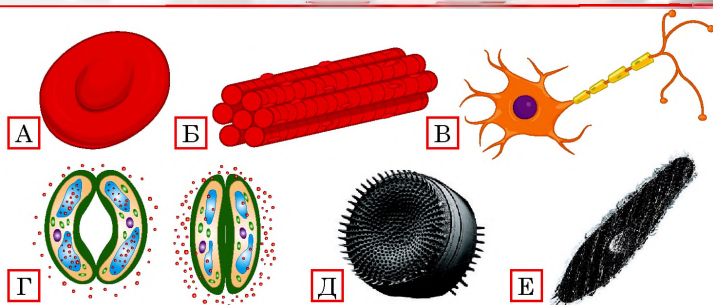
Рис. 1.3. Різноманітність клітин
