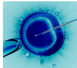
Рис. 44.3. Екстракорпоральне запліднення
