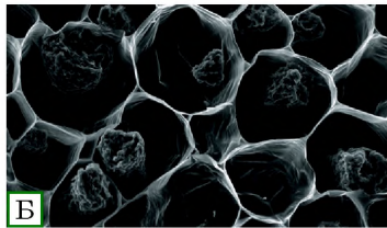
Рис. 9.6. Мікориза
