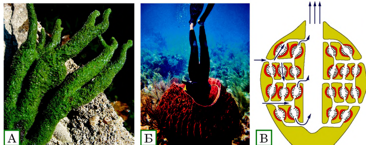
Рис. 10.1. Губки
