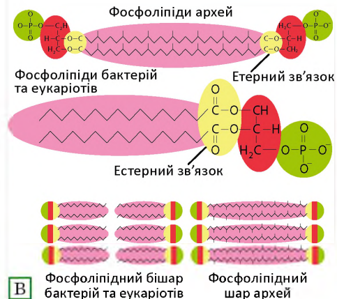
Рис. 5.7. Археї
