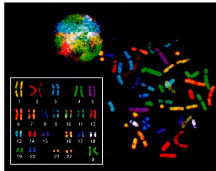
Рис. 30.4. Каріотип людини
