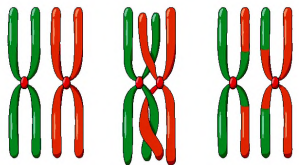
Рис. 31.2. Схема кросинговеру
