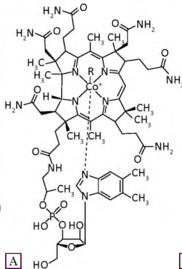
Рис. 18.3. Вітамін B_{12}
