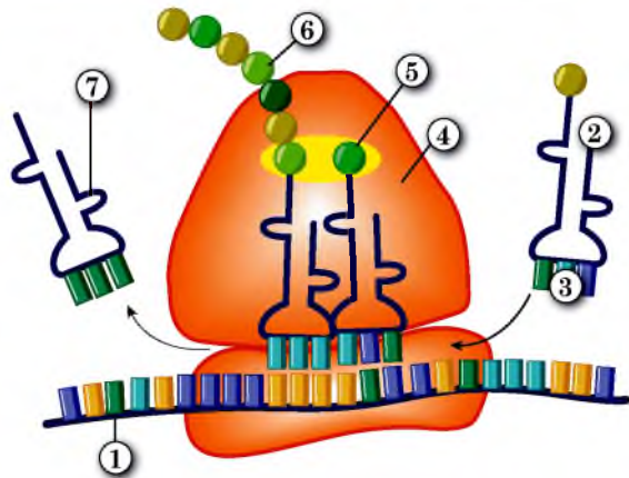
Рис. 29.2. Схеми трансляції
