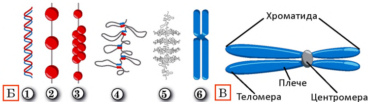
Рис. 30.2. Організація хроматину
