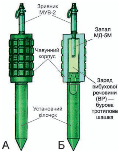
Іл. 23.3. Противіхотна осколкова міна ПОМЗ-2М А — загальний вигляд; Б — повздовжній розріз
