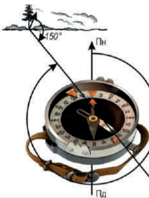
Іл. 32.1. Визначення магнітного азимута
