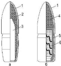
Іл. 22.4. Куля: а — звичайна зі сталевим осердям; б — трасуюча; 1 — оболонка; 2 — свинцева сорочка; 3 — сталевга серцевина; 4 — свинцева серцевина; 5 — стаканчик трасера; б — трасуюча суміш
