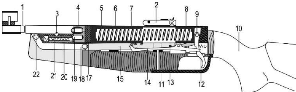
Іл. 20.4. Складові частини і механізми рушниць ІЖ-38: 1 — ствол; 2 — приціл; 3 — вісь ствола; 4 — прокладка ствола; 5 — коробка ствола; 6 — поршень; 7 — пружина бойова; 8 — колодка механізму спускового; 9 — штифт колодки; 10 — ложа; 11 — гвинт ложі задній; 12 — гачок спусковий; 13 — шептало; 14 — важіль блокування; 15 — важіль зведення; 17 — манжета; 18 — шарнір; 19 — клин; 20 — ригель; 21 — пружина ригеля; 22 — вісь шарніра
