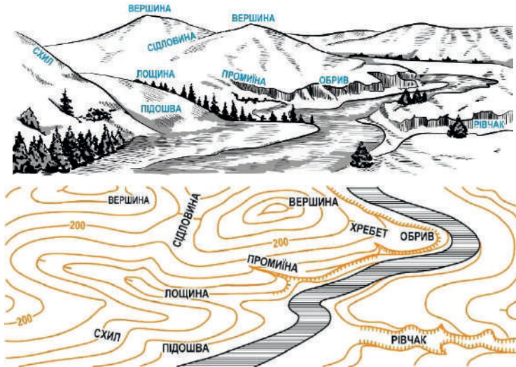
Іл. 33.2. Зображення рельєфу місцевості горизонталлями
