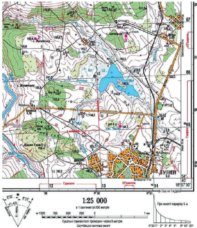
Іл. 34.3. Визначення прямокутних координат за топографічною картою
