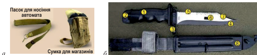
Лл. 18.4. Комплект для автомата Калашнікова: а — сумка для магазинів, пасок для носіння автомата; б — багнет-ніж: 1 — ручка; 2 — кнопка фіксатора; 3 — кільце; 4 — лезо; 5 — шилка; 6 — отвір; 7 — ріжуча грань; 8 — піхви
