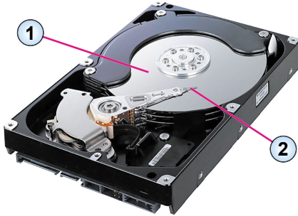
Мал. 2.6. Будова накопичувача на жорстких магнітних дисках
