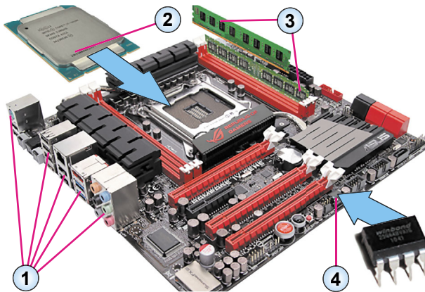
Мал. 2.4. Материнська плата комп'ютера
