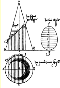
Спосіб побудови еліпса як перетину конуса, кресляр Альбрехт Дюрер, 1525 р.
